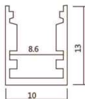
524- Mini Profile
