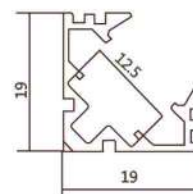
504 CORNER 19×19
